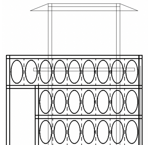
櫓側面
